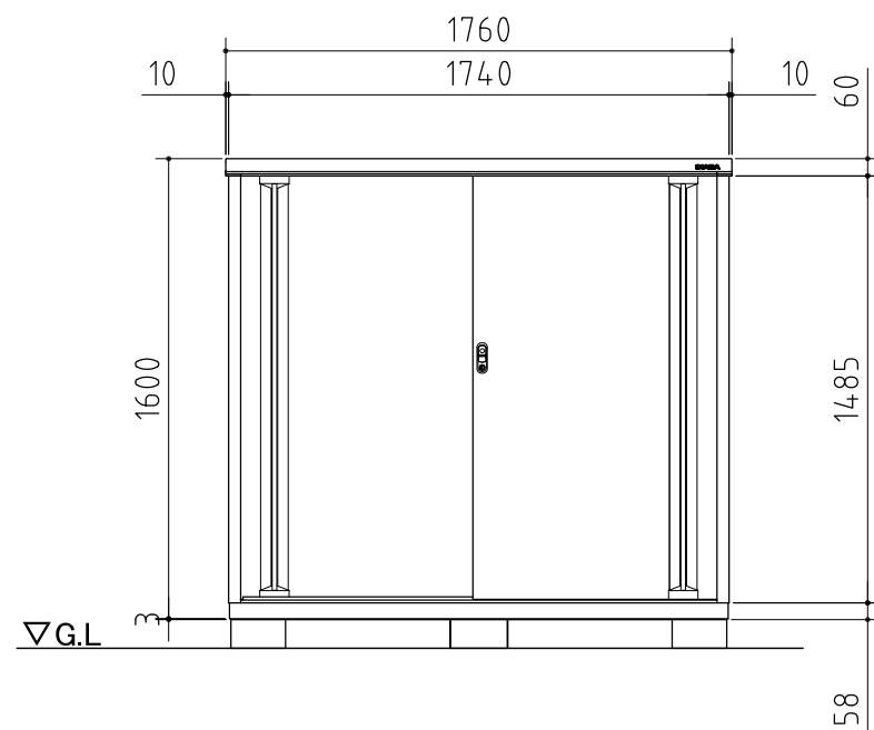
正面図
